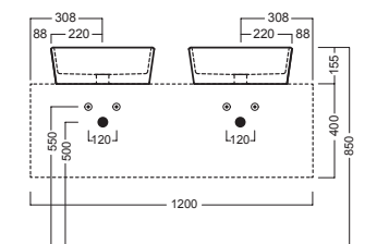
SLIDING wood system_taglio 4 doppio - cut 4 double
