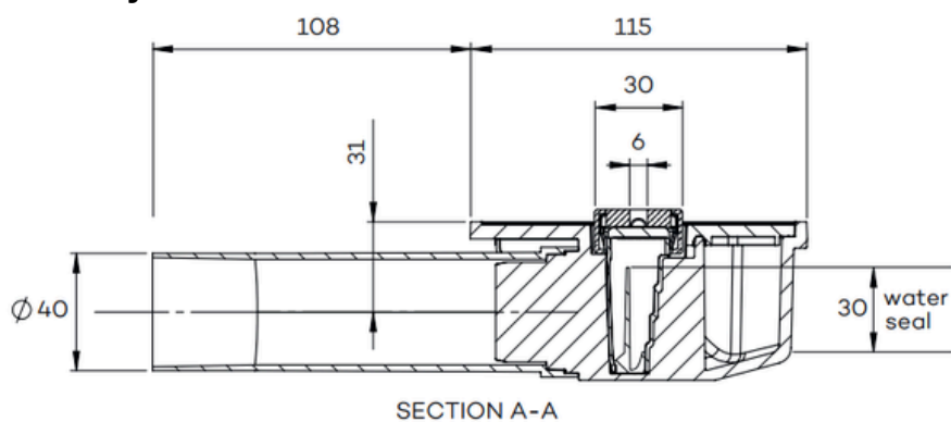
Zijaanzicht
