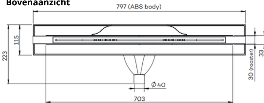
Bovenaanzicht
