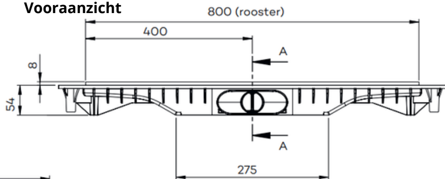
Vooraanzicht
